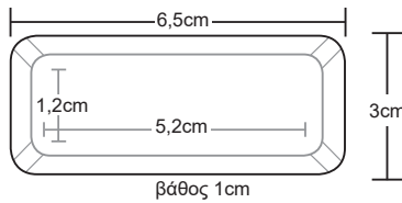
Λαμαρίνα αλουμινάτε για κεκάκια Aluminium sheet for cakes
